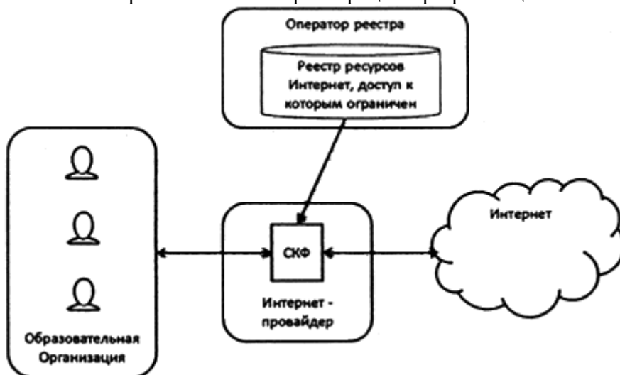
Рис.4. Схема работы контент-фильтрации при размещении у интернет-провайдера
